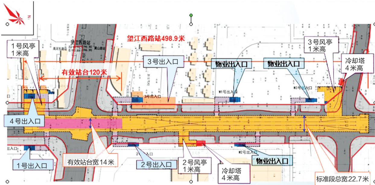
望江西路站近期总平面图
