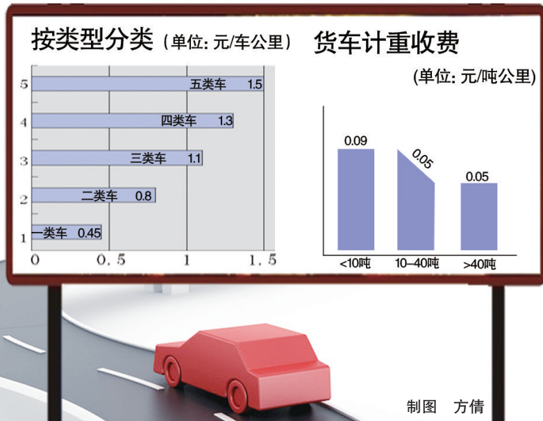
高速公路收费基本费率标准(调整后)
